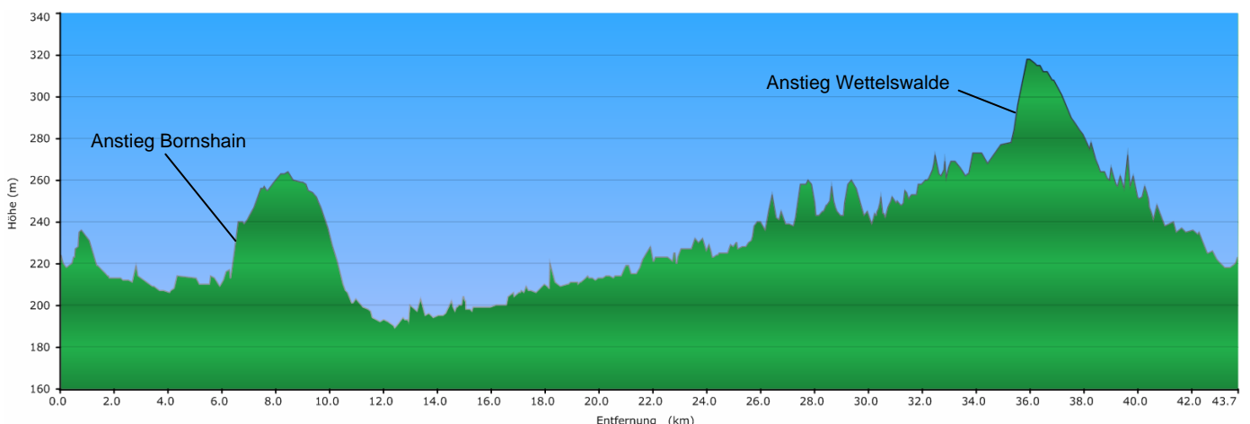
Höhenprofil zwischen 189 Hm und 318 Hm
